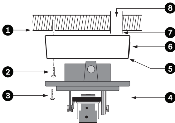
Рисунок 3.7 Установка на поверхность - заднее соединение
