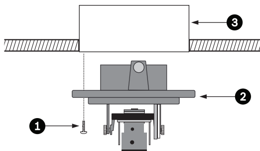
Рисунок 3.4? Утопленный монтаж - распределительная коробка (4S)
