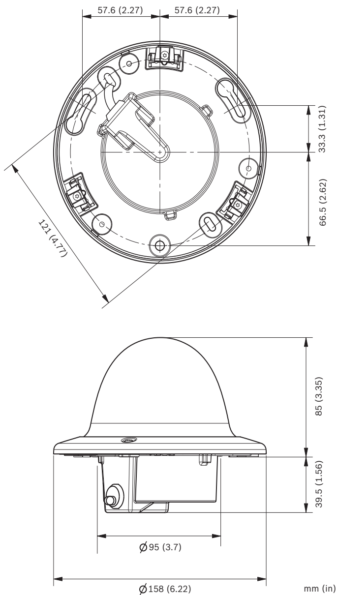
Рисунок 8.1 Размеры - уплотненный монтаж
