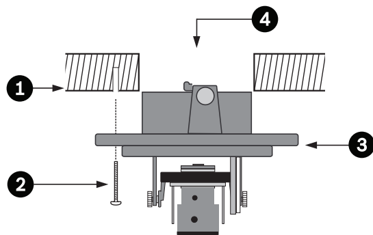
Рисунок 3.3.2 Утепленный монтаж - полая поверхность
