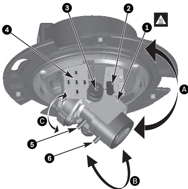
Рисунок 4.1 Детали камеры
